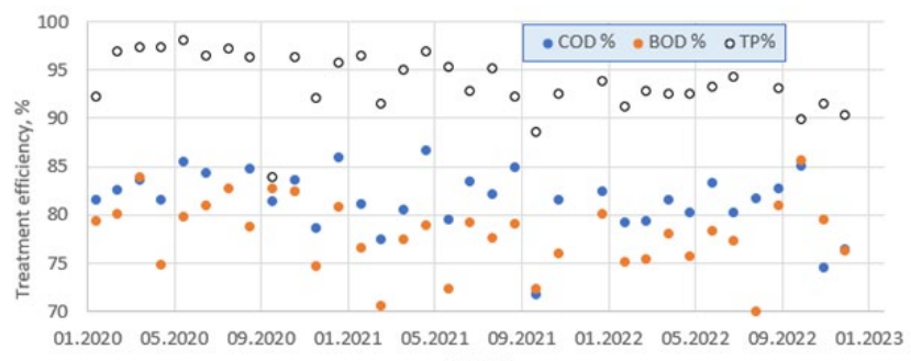
Figur 1. Fjerning av KOF, BOF og Total-P ved SFR i 3 år med super-optimalisert koagulering.
