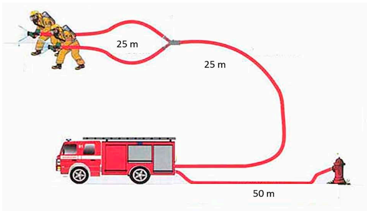
Figur 37: Eksempel på slokkeoppsett for å unngå uhensiktsmessig kort avstand mellom brannkummer eller hydranter.
