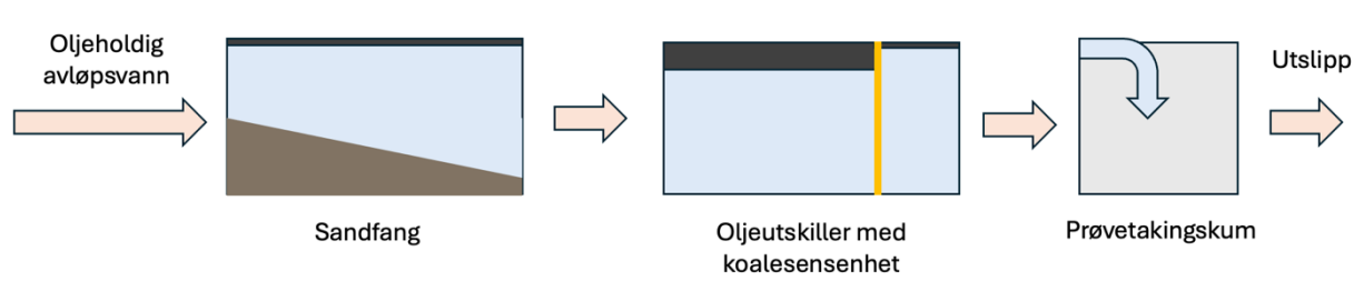
Figur 4. Skjematisk oppbygging av et oljeutskilleranlegg
